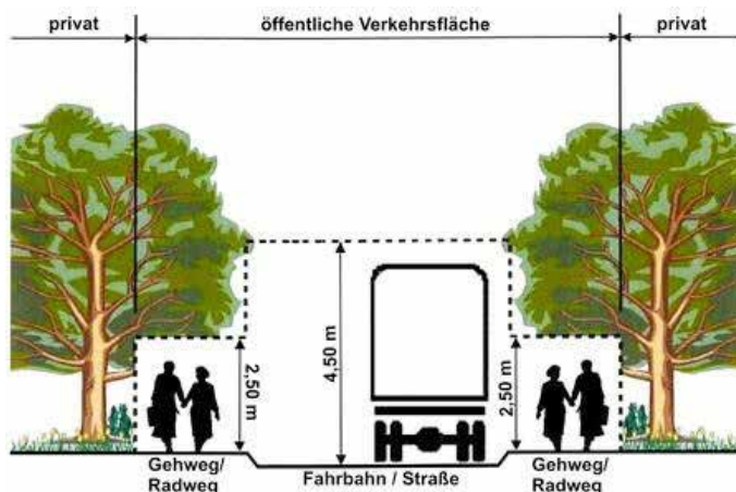
Lichtraumprofil
