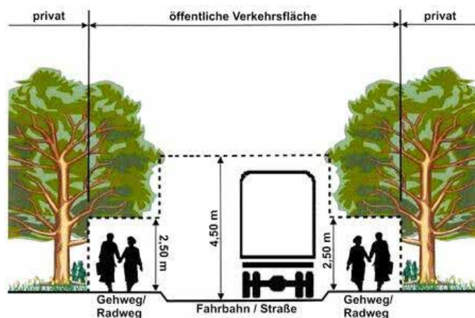
Lichtraumprofil
